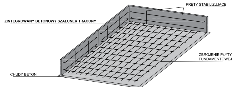
Szalunek tracony do płyty fundamentowej
