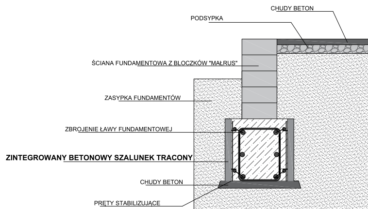
Szalunek tracony do ław fundamentowych
