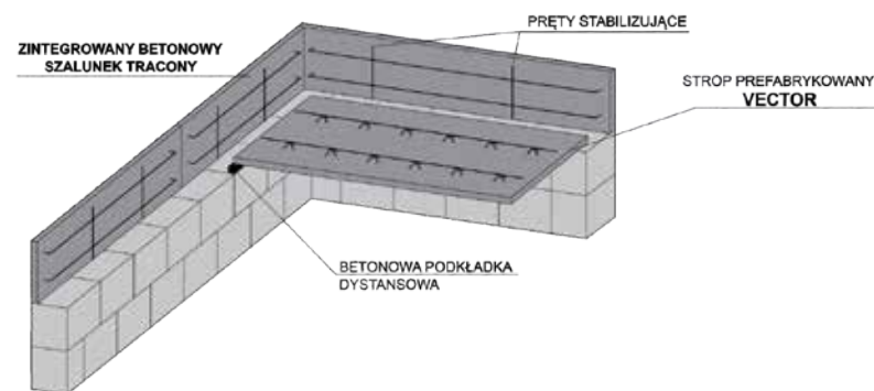
Tracone deski szalunkowe dla stropów
